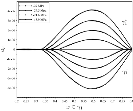
а) Значение функции u_\nu на \gamma_1^\pm
