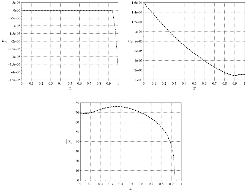
Рис. 2 — Значение функций u_n , u_\tau , |\sigma_n| на \Gamma_2 для II примера
