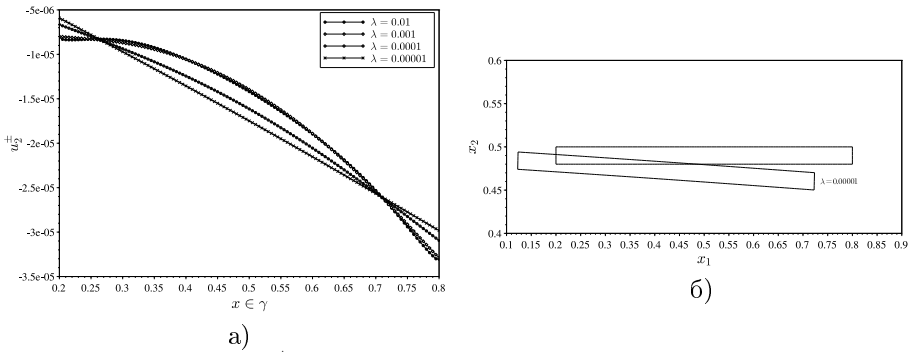
Рис. 7 — Значения u_2^\pm на трещине и перемещение жёсткого включения
