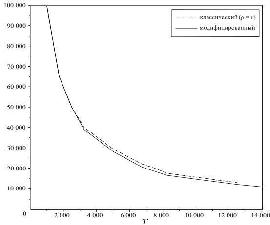
Рис. 5 — Количество итераций по двойственной переменной в зависимости от параметра r .
