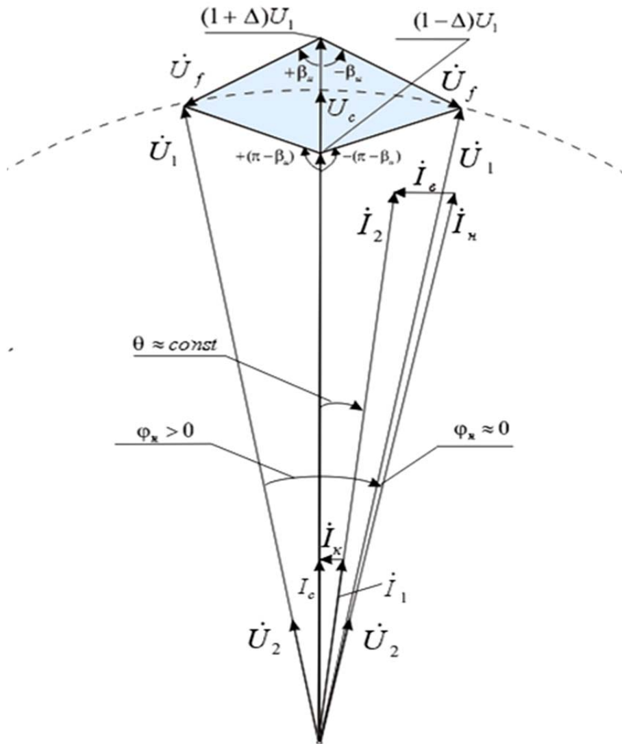
Рисунок 4. Векторная диаграмма напряжений и токов силового трансформатора подстанции с КРМЧН
