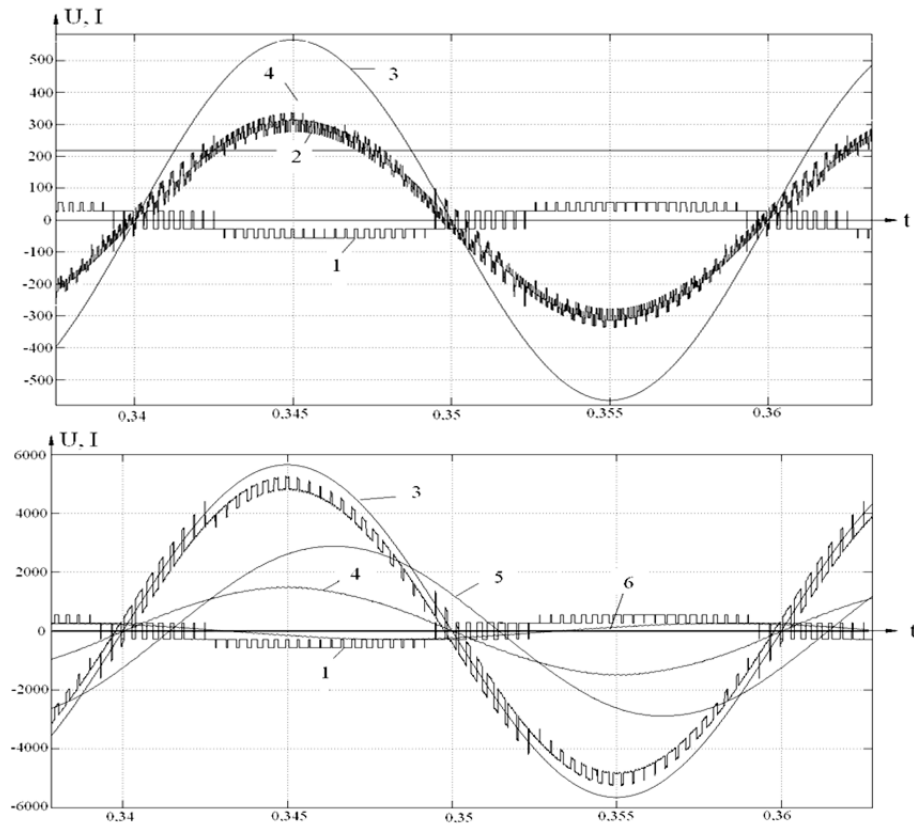
Рисунок 19. Осциллограммы системы КРМЧН-ТП при повышенном напряжении в сети и RL-нагрузке подстанции (масштаб относительный): 1 – напряжение вольтодобавки; 2 – напряжение нагрузки; 3 – напряжение сети; 4 – ток сети; 5 – ток нагрузки; 6 – ток на входе управляемого выпрямителя.
