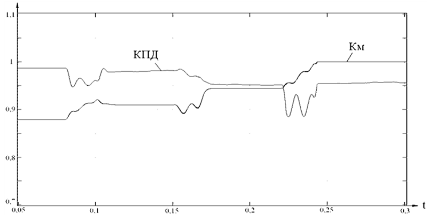
Рисунок 20. Графики мощностей (сверху) и энергетических показателей (снизу): 0,08с - включен управляемый выпрямитель; 0,15с – включен инвертор напряжения; 0,22с – включена батарея косинусных конденсаторов.
