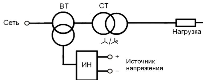
Рисунок 8. Схема для исследования инвертора при работе на ВТ
