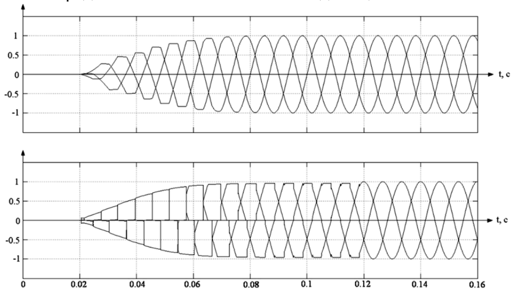
Рисунок 16. Осциллограммы трехфазных напряжений (сверху) и токов (снизу) конденсаторов при пуске
